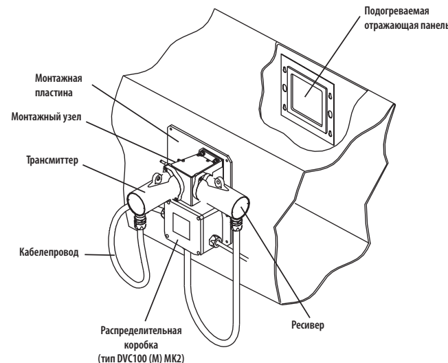
Разводка кабелей трансмиттера детектора с поперечно-проходной схемой
