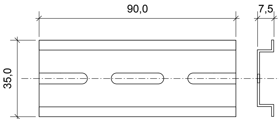
Стандартная монтажная планка (№ по каталогу 9602.0050.10.03)
