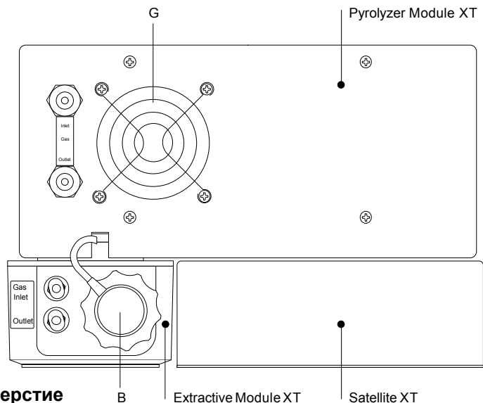
Рисунок 3: Вид всей системы сверху
