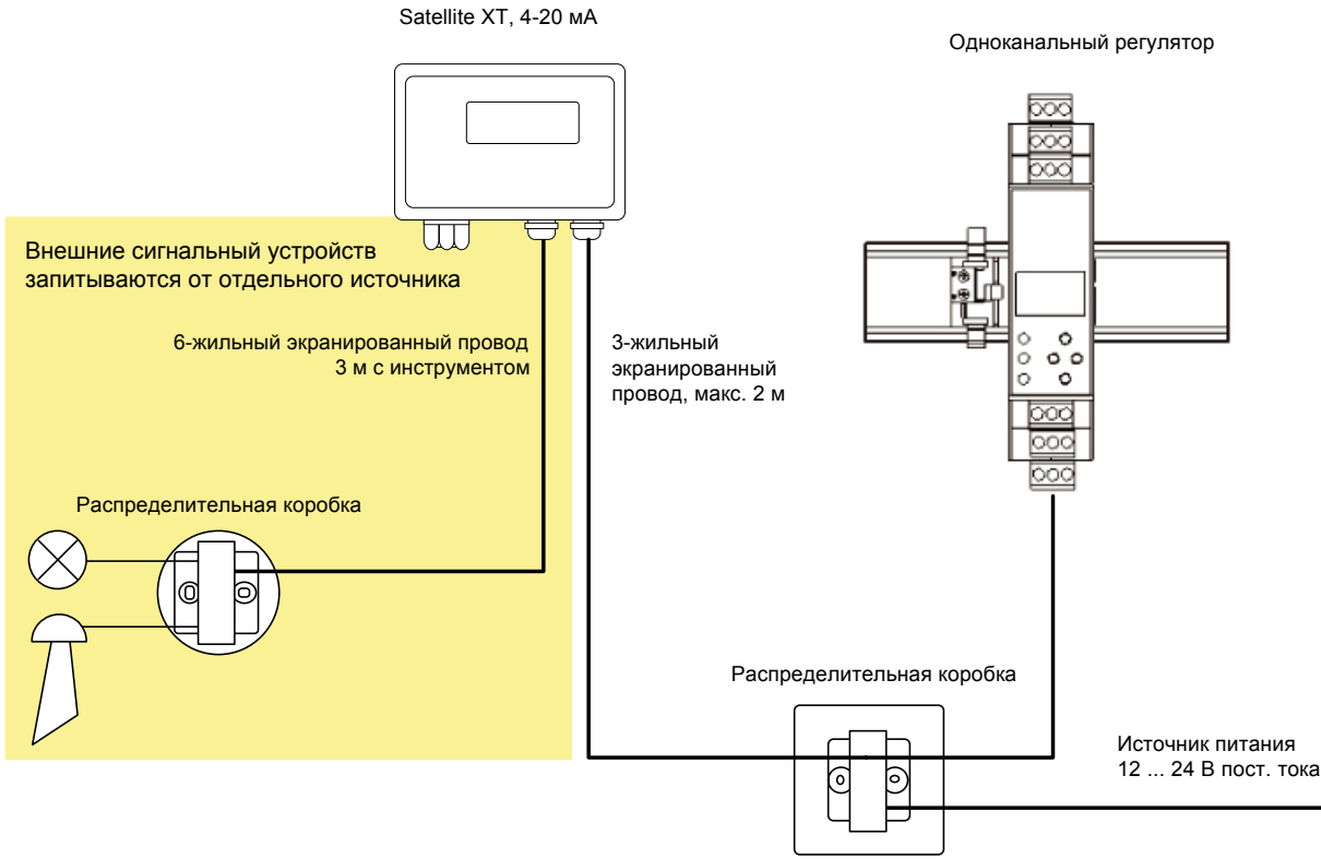
Схема проводки Satellite XT 4-20 мА, одноканальный регулятор
