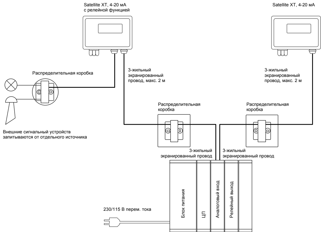
Схема подключения Satellite XT 4-20 мА и программируемого логического контроллера (ПЛК)
